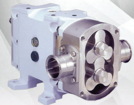
مضخة لوب
