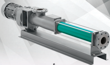
مضخة أحادية
