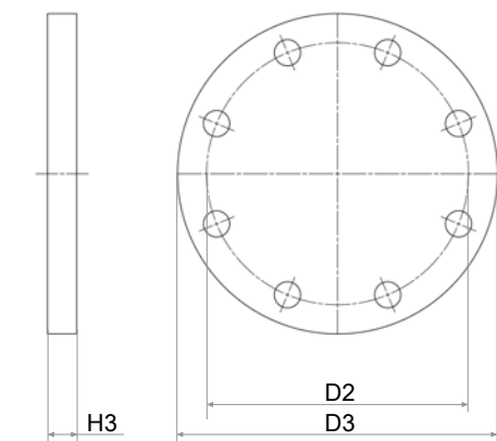
Blank flange
