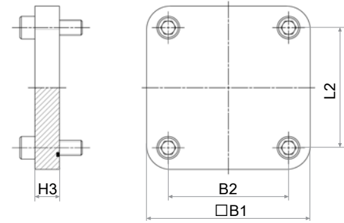
Blank flange
